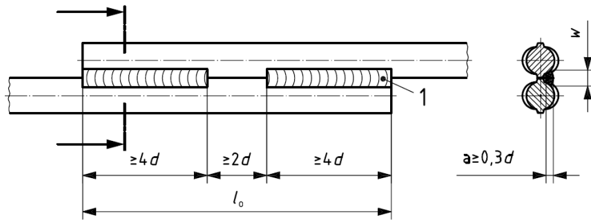
Figure 1 — Assemblage à recouvrement
