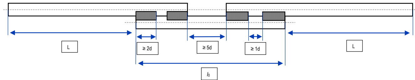
Figure 1 — Assemblage à recouvrement
